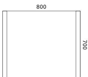
VIA VALOPEILI 80X70 • mitat L800 x K700 x S60 mm
